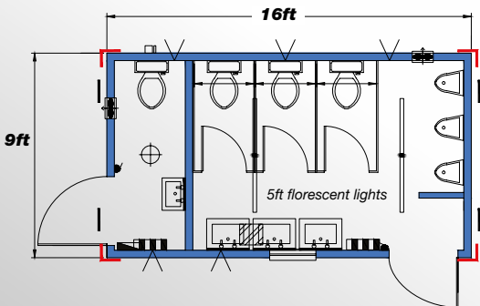
3 + 1 Toilet - 16ft x 9ft
