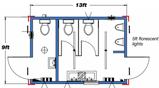
2 + 1 Toilet - 13ft x 9ft
